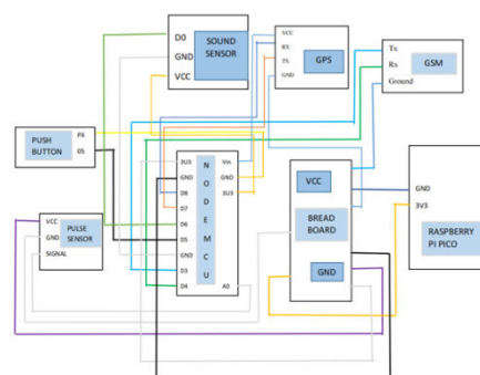
Figure 3 :Circuit Diagram
